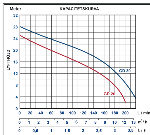
GD20A/ GD30A
