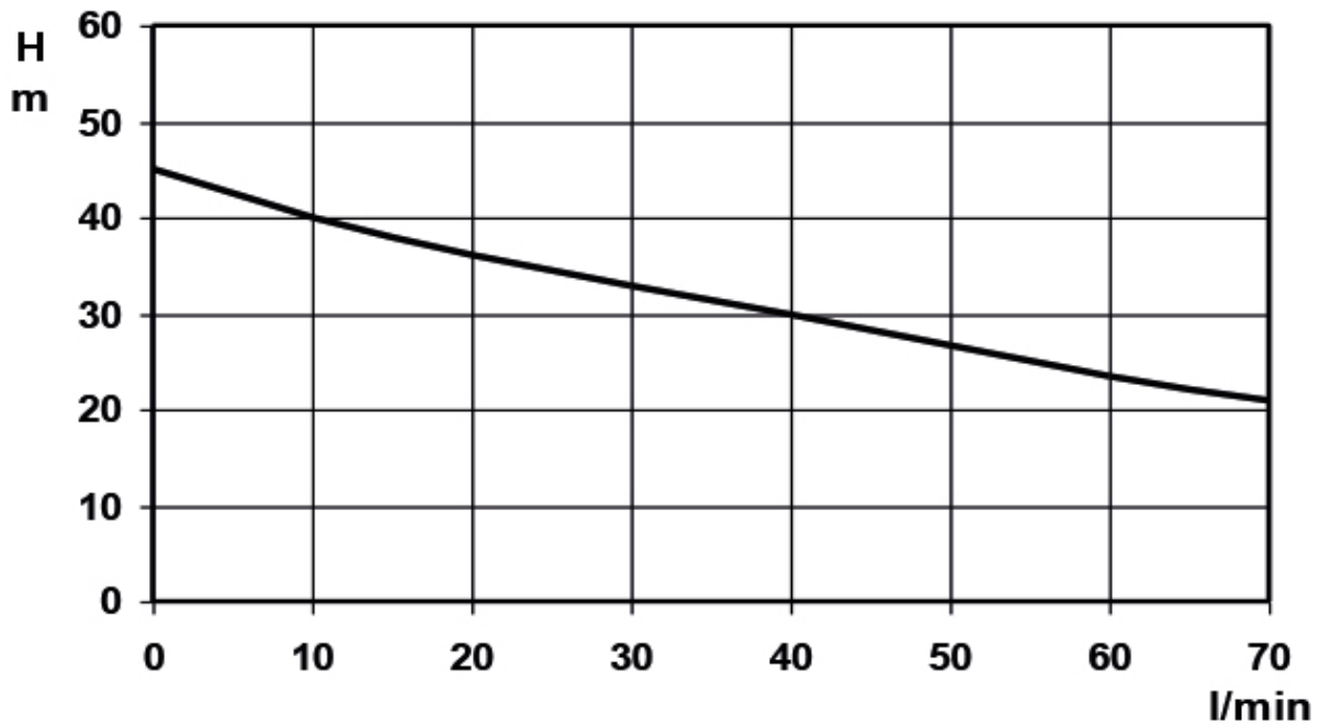
Kapacitetskurva
