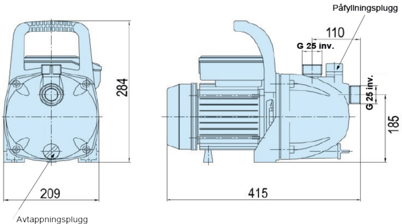
Måttskiss
