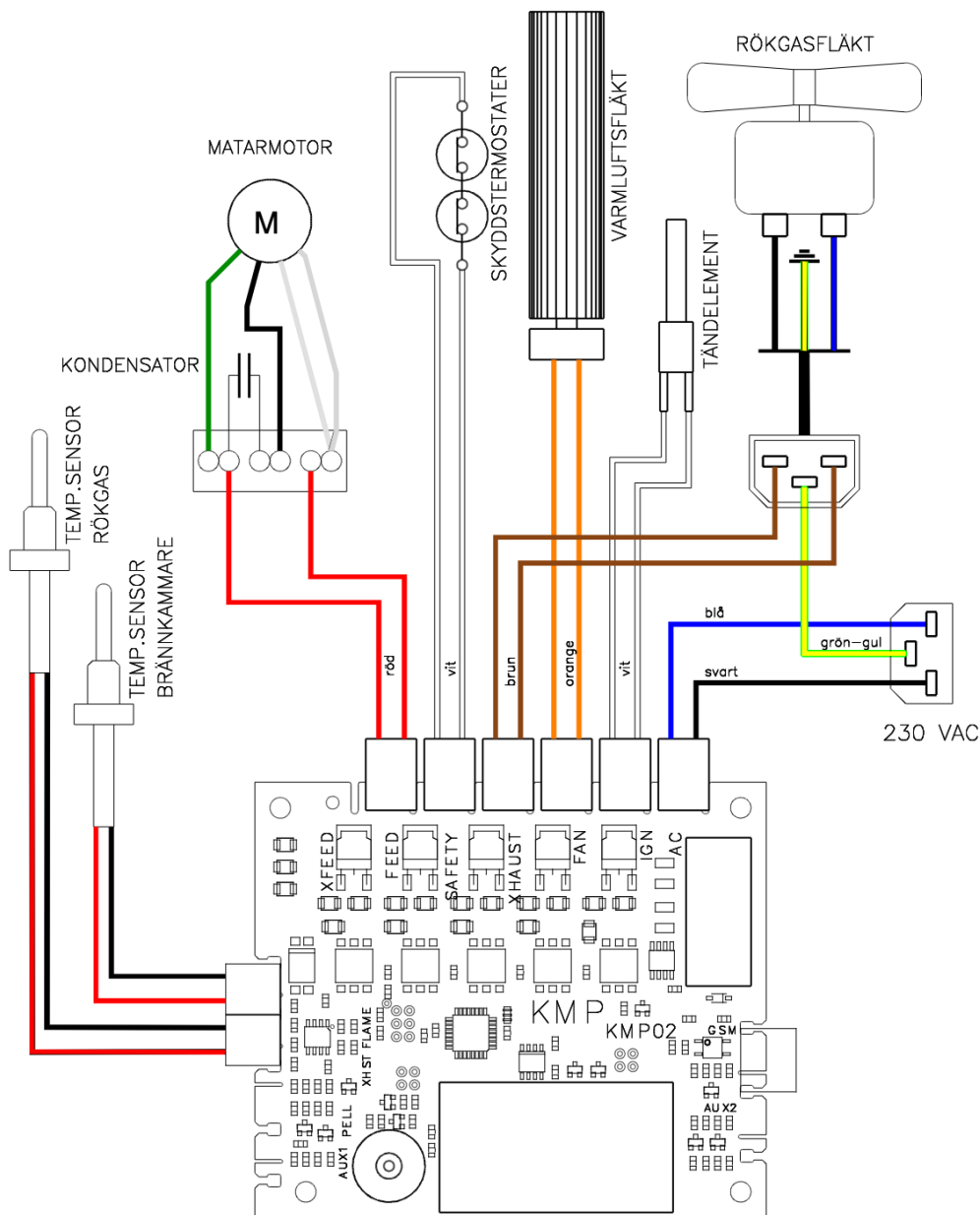
Kopplingsschema
